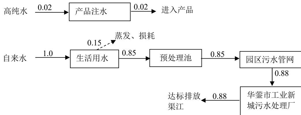
图 2-1 项目水量平衡图 单位 \text{m}^3/\text{d}
